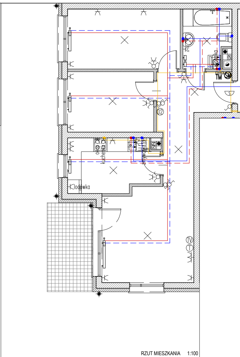
RZUT MIESZKANIA 1:100
