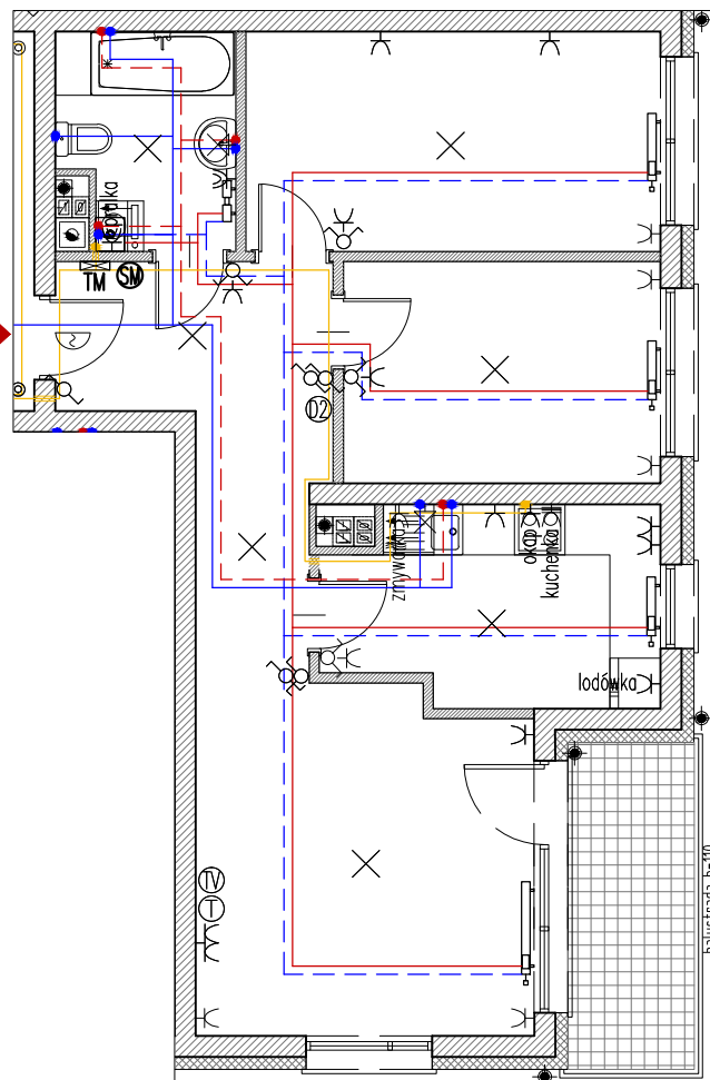
RZUT MIESZKANIA 1:100
